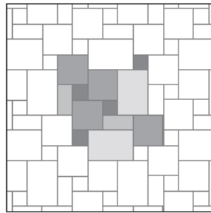
Layout 2 600×900: 33,3% 600×600: 44,5% 300×600: 11,1% 300×300: 11,1%
