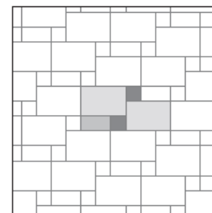
Layout 5 600×900: 75% 300×600: 12,5% 300×300: 12,5%
