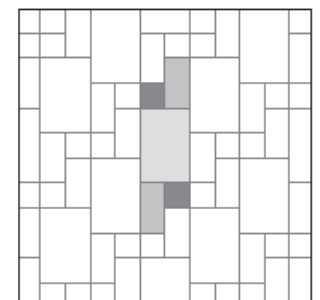
Layout 6 600×900: 50% 300×600: 33,4% 300×300: 16,6%
