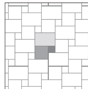
Layout 4 600×900: 54,5% 600×600: 36,5% 300×300: 9%
