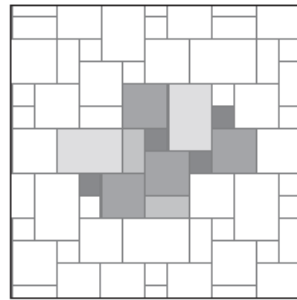
Layout 3 600×900: 33,3% 600×600: 44,5% 300×600: 11,1% 300×300: 11,1%
