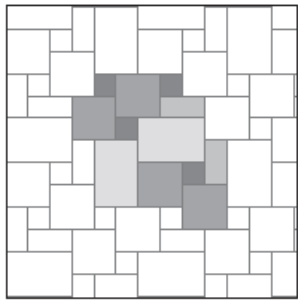
Layout 1 600×900: 33,3% 600×600: 44,5% 300×600: 11,1% 300×300: 11,1%
